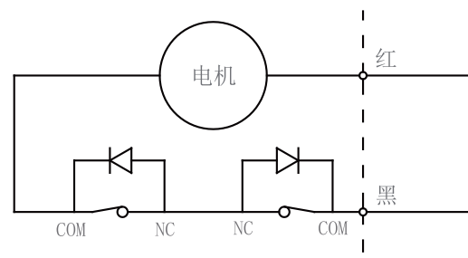
霍尔信号反馈电机内部接线方式
